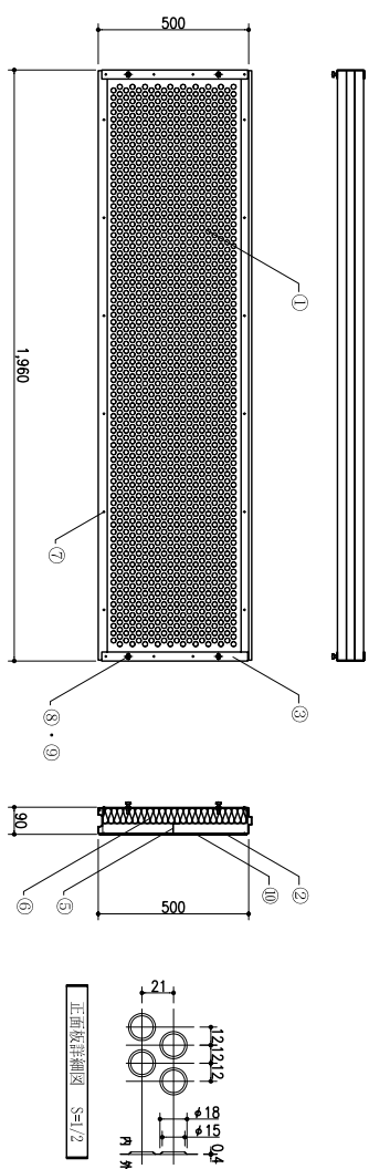
フェニクスカーン防音パネルBP-90 詳細図
