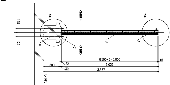
フェニクスカーン防音パネルBP-90 詳細図
