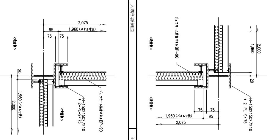
フェニクスカーン防音パネルBP-90 詳細図
